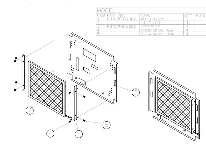
FIGURE 5-4: DISPLAY PAC-PPC 15.1" LCD MODULE
