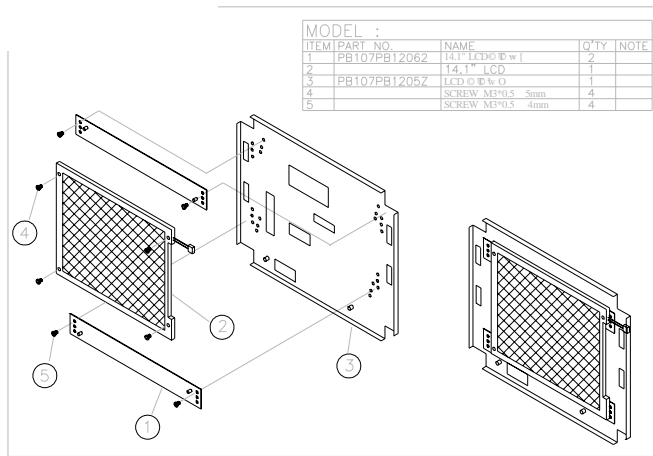
FIGURE 5-3: DISPLAY PAC-PPC 12.1" LCD MODULE
