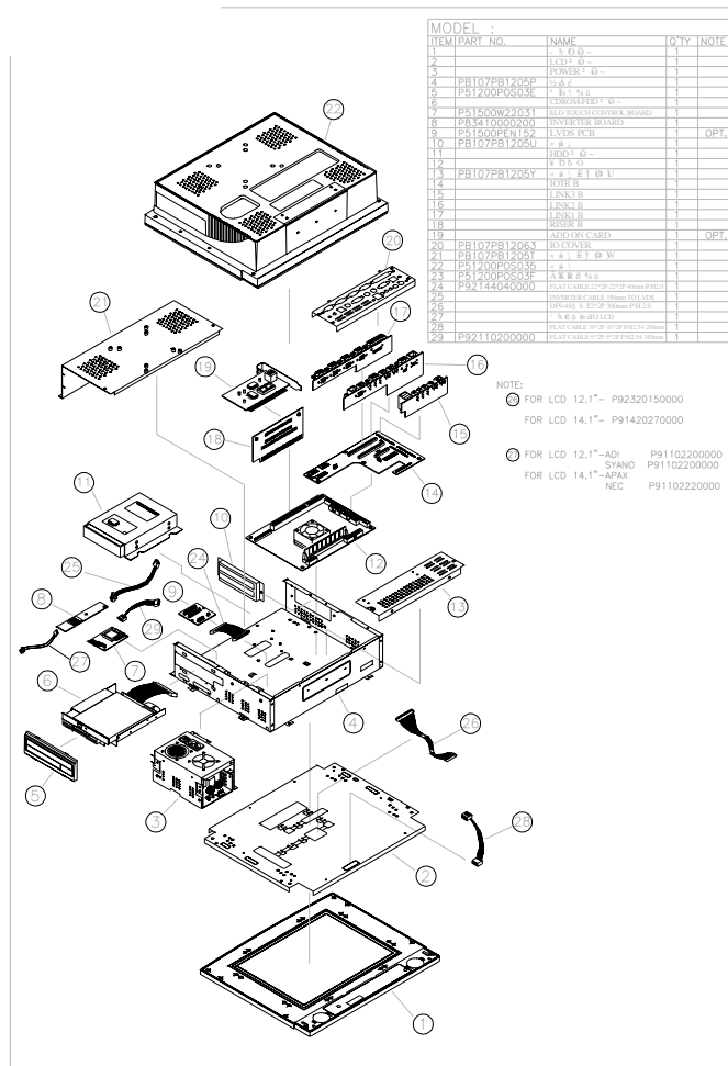
FIGURE 5-1: DISPLAY PAC-PPC EXPLODED
